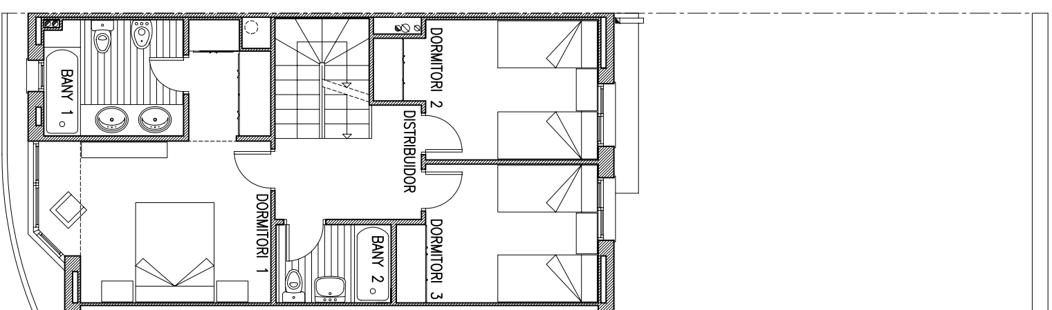
PLANTA PIS
