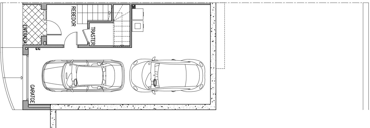
PLANTA SEMISSOTERRANI
