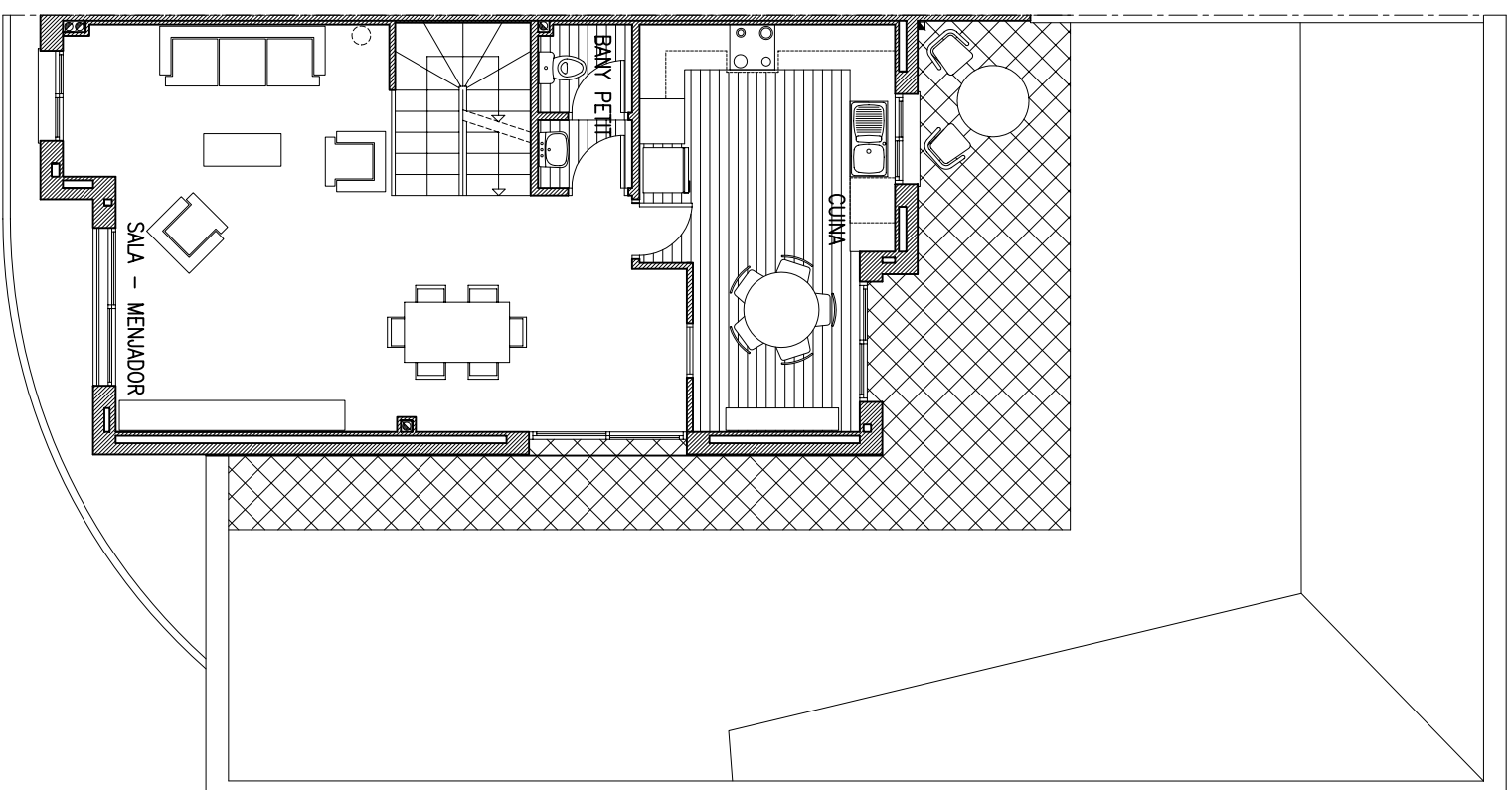
PLANTA BAIXA
