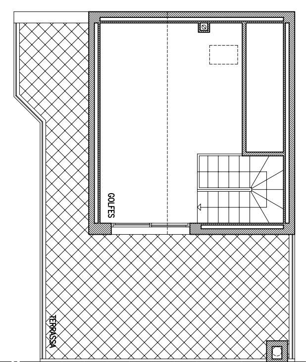
PLANTA PIS
