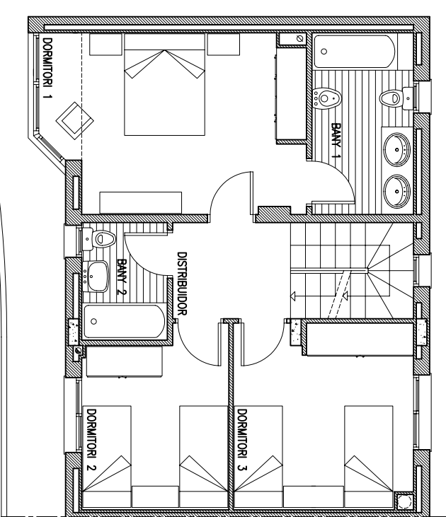
PLANTA PIS
